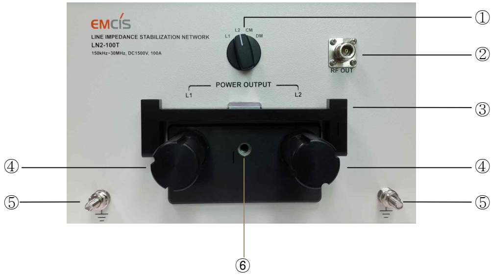
그림1. 전면패널
